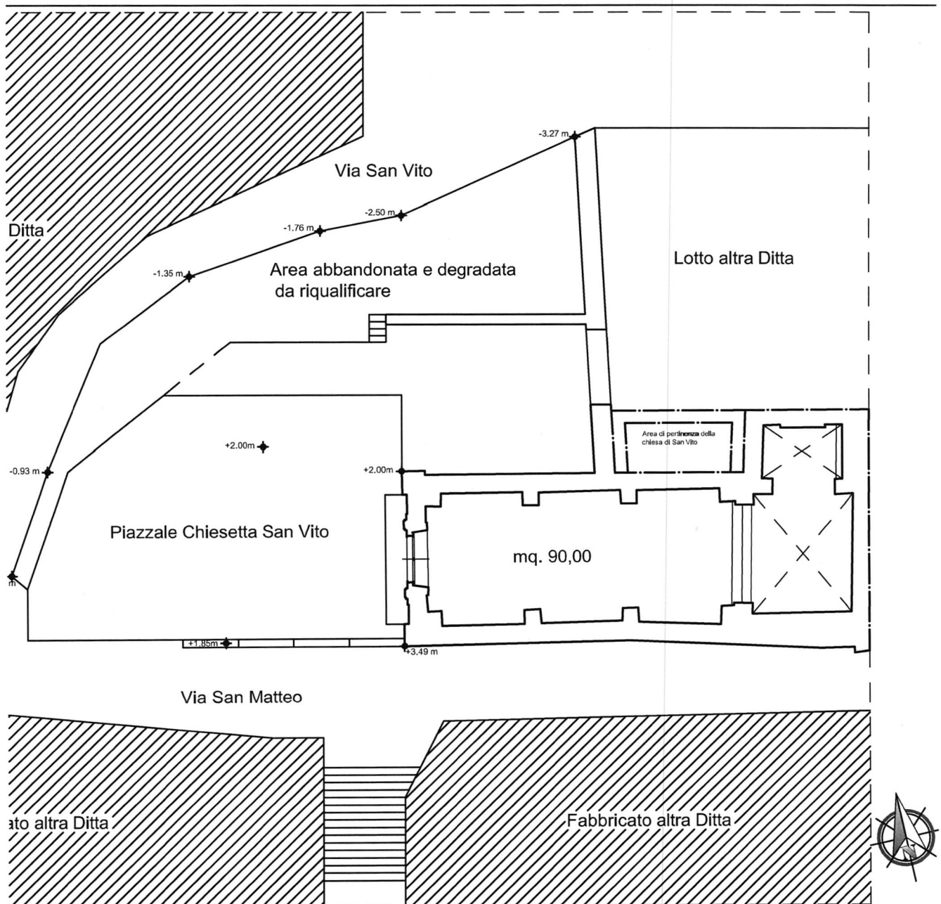
Planimetria scala 1:200
