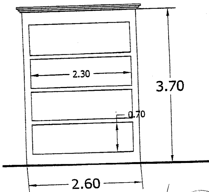
Prospetto Frontale
