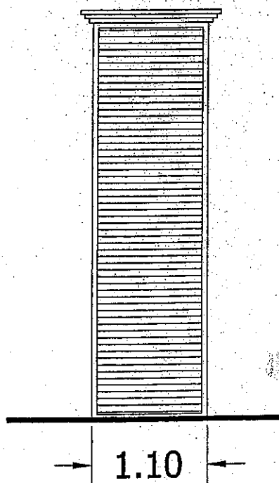
Prospetto Laterale
