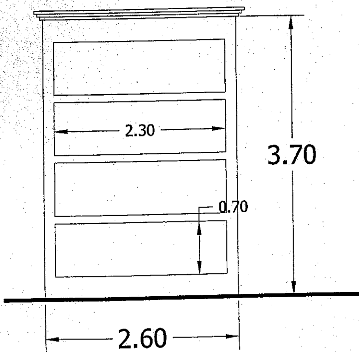
Prospetto Frontale
