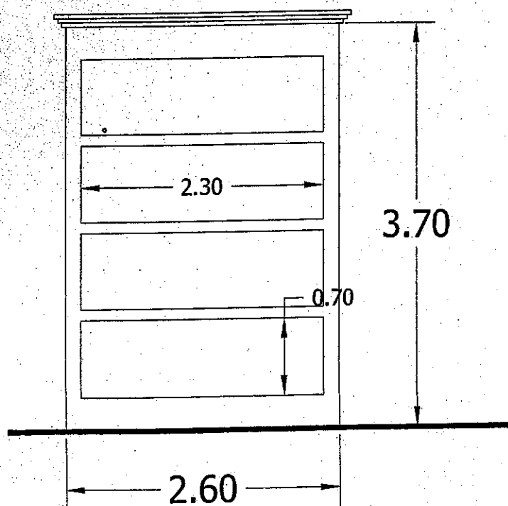
Prospetto Frontale
