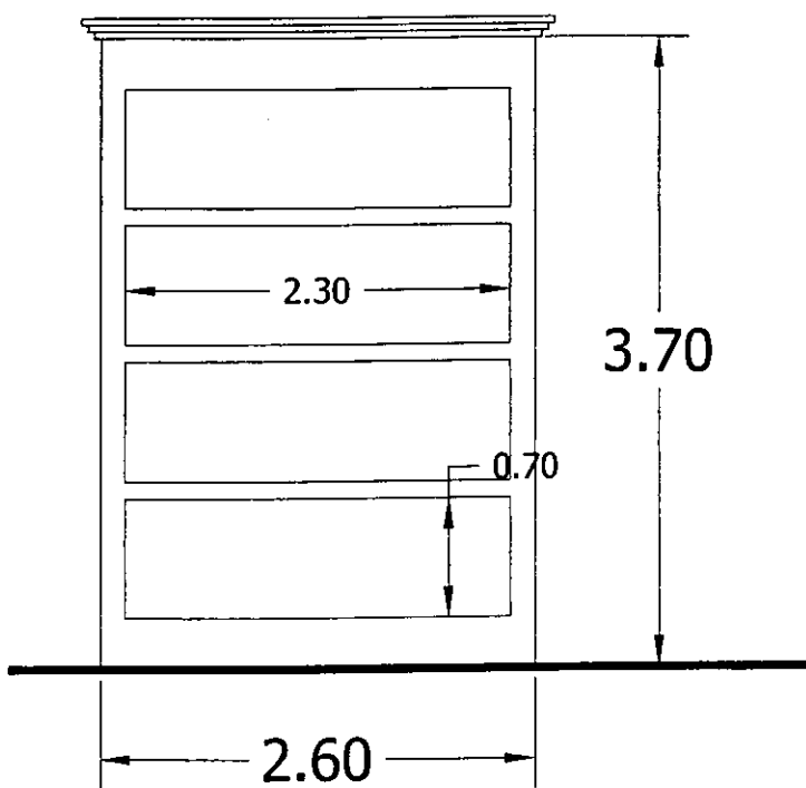
Prospetto Frontale
